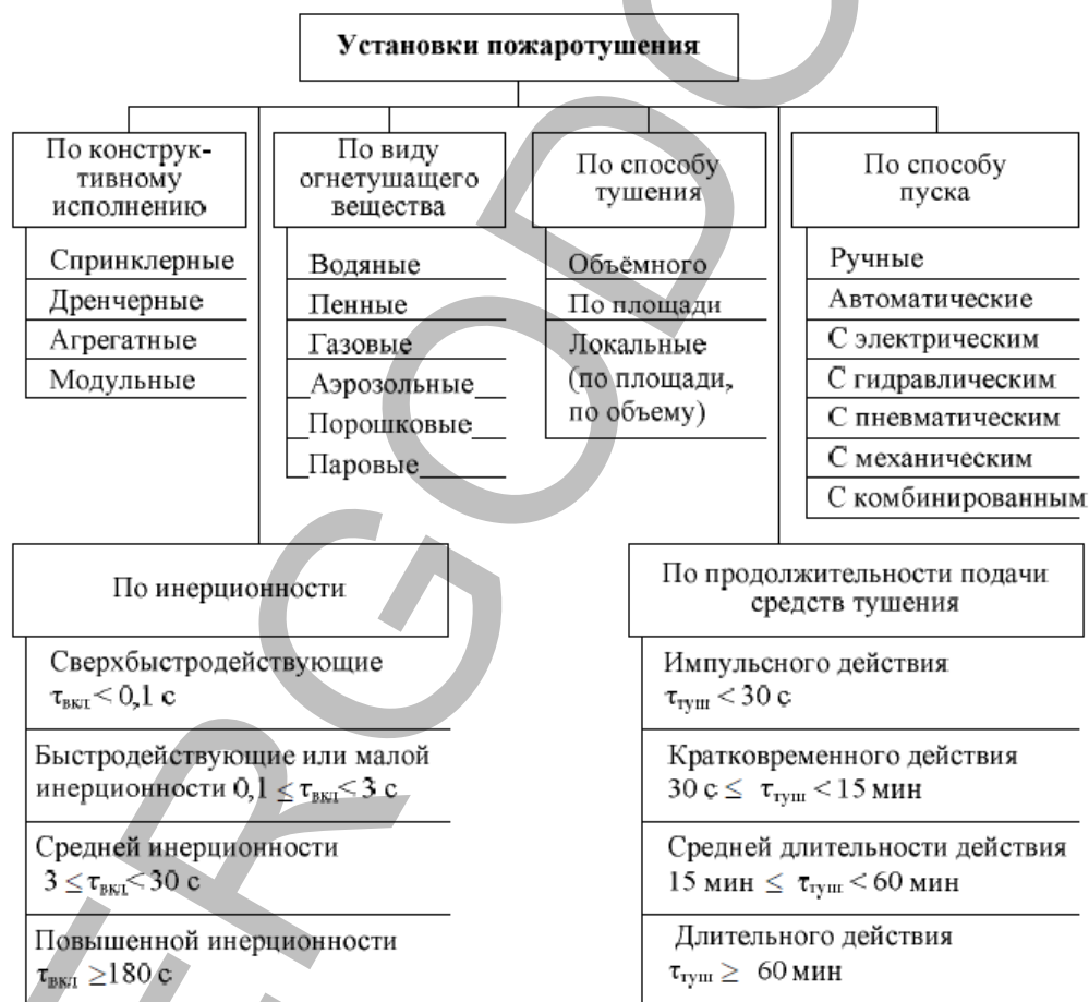
Рис. 1.1. Обобщенная классификация установок пожаротушения
