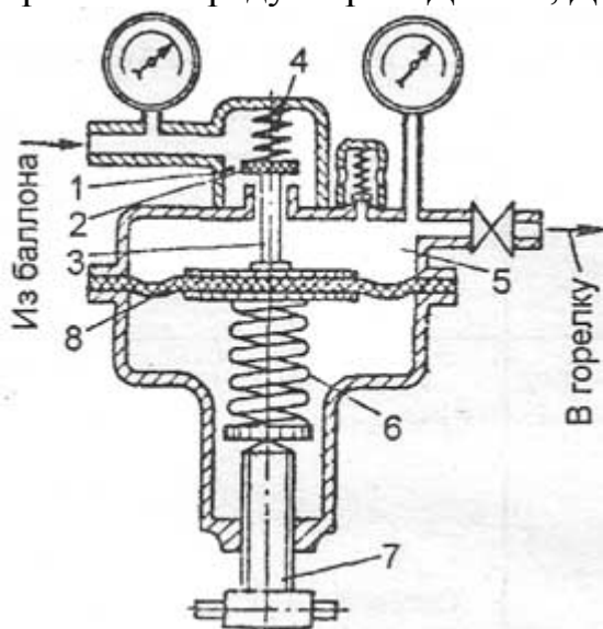
Рис. 1. Схема устройства однокамерного редуктора
