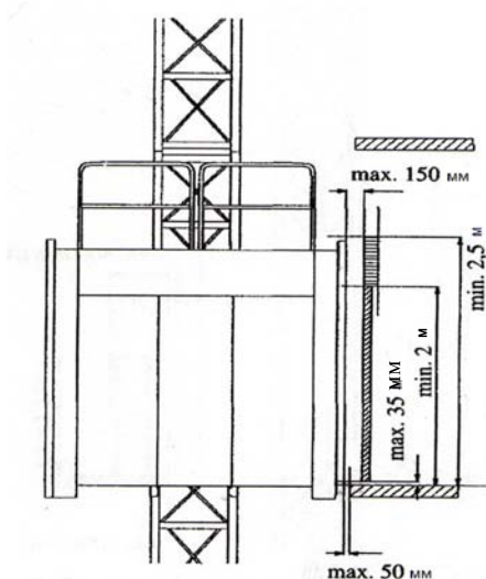
Рисунок 5 – Пример дверей погрузочной площадки
